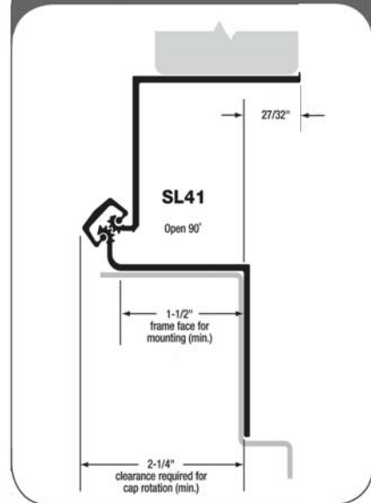
Fig. 2 Door Open 90°
