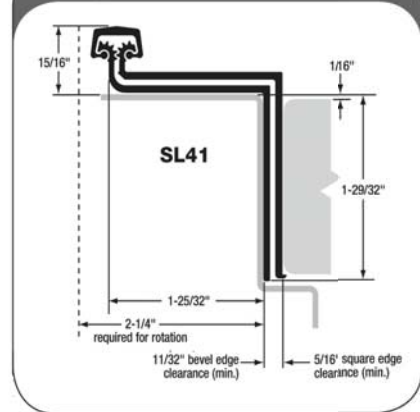
Fig. 2 Door Open 90°
